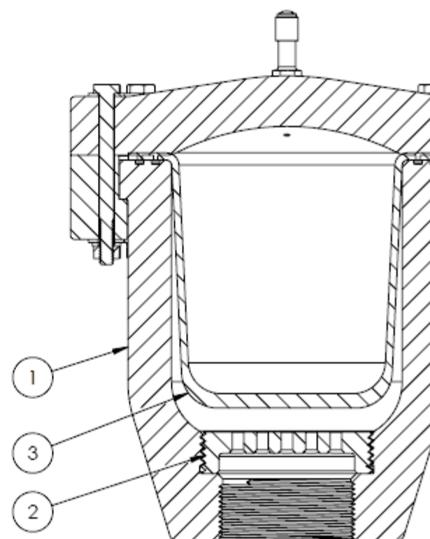
SECTION A-A
